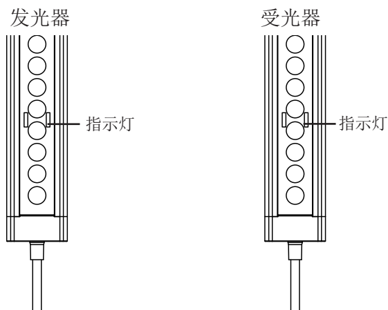
图4-2 MCI系列安全光幕指示灯图
