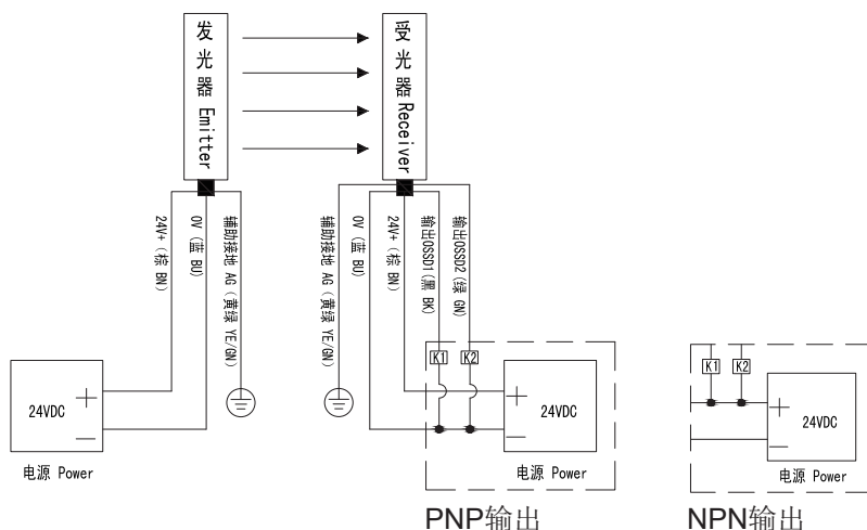
图 6-1 MCI 系列安全光幕接线图
