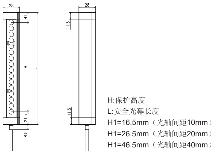
图4-3 MCI系列安全光幕外形尺寸图
