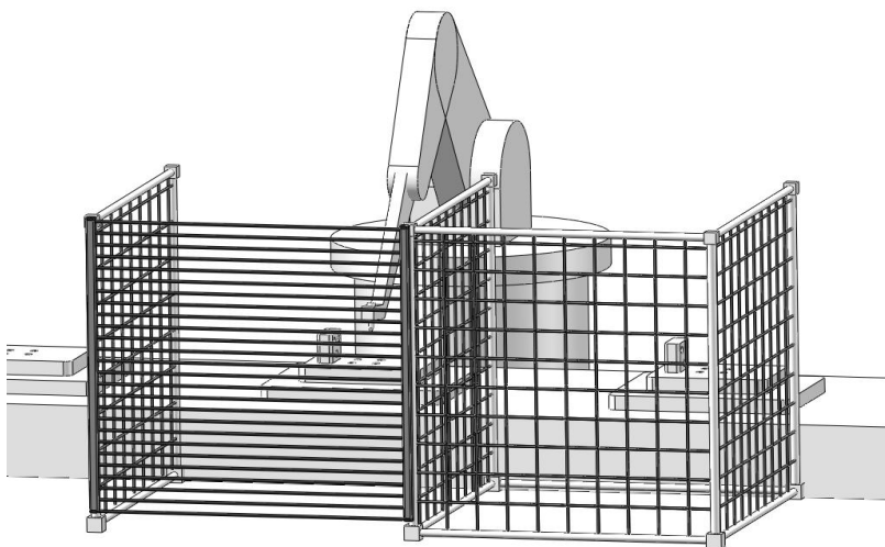
图3-6 使用MCI系列安全光幕的进入保护
