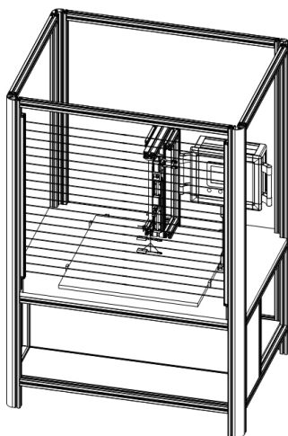
图3-4 使用MCI系列安全光幕的危险点保护
