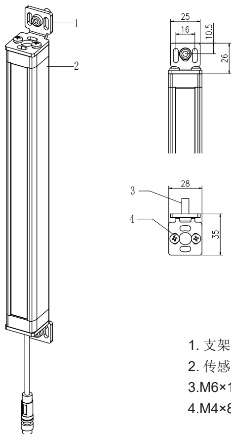
图5-5 正装/侧装支架安装示意图
