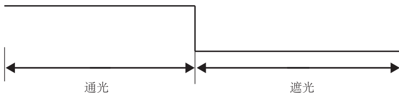
图 6-5 PNP 输出的 MCI 系列安全光幕波形图
