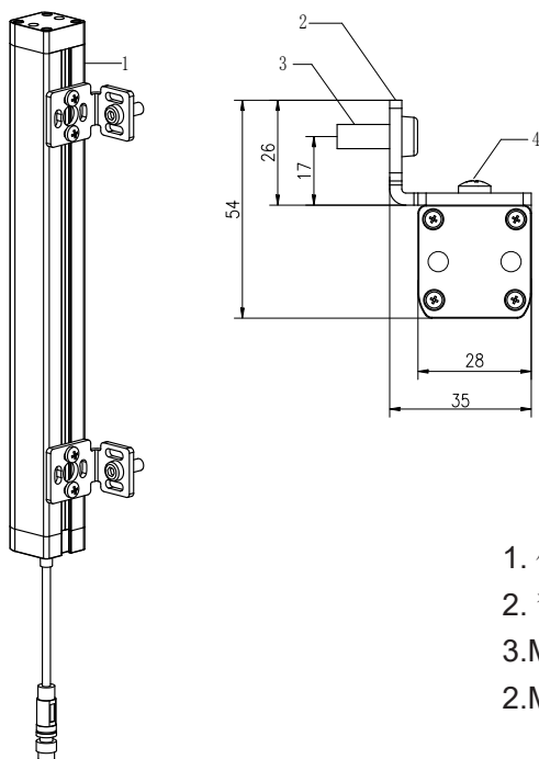
图5-6 弯角支架安装示意图
