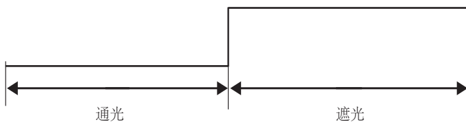
图 6-4 NPN 输出的 MCI 系列安全光幕波形图
