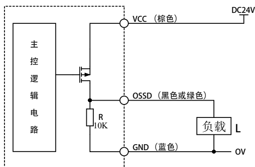
图 6-3 MCI 系列安全光幕 PNP 输出结构图
