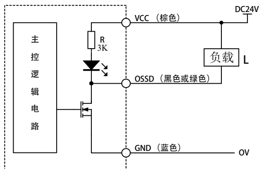
图6-2 MCI系列安全光幕NPN输出结构图
